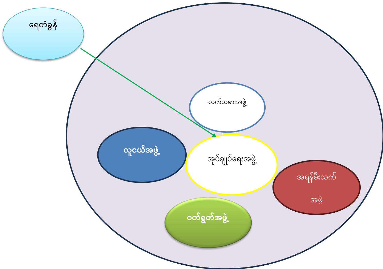
Venn Diagram
